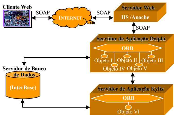
FIGURA 4 ARQUITETURA DO WEBCELLP.
