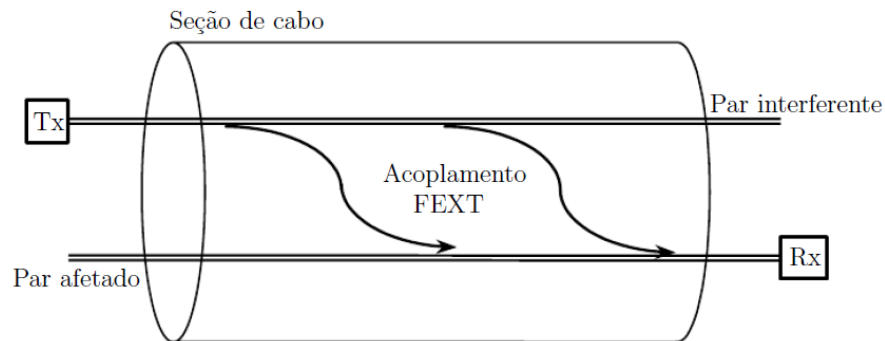
Figura 2.4: Acoplamento FEXT.
